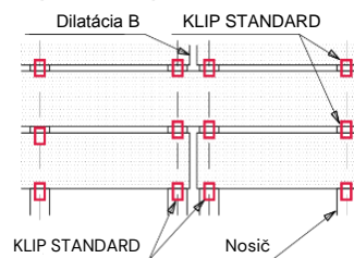
Obr. 5 Napájanie terasových dosiek pomocou KLIPU STANDARD
